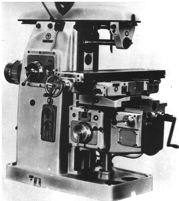
Универсална фрезова машина ФУ250
